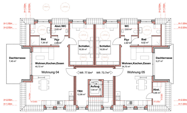
GRUNDRISS DG
