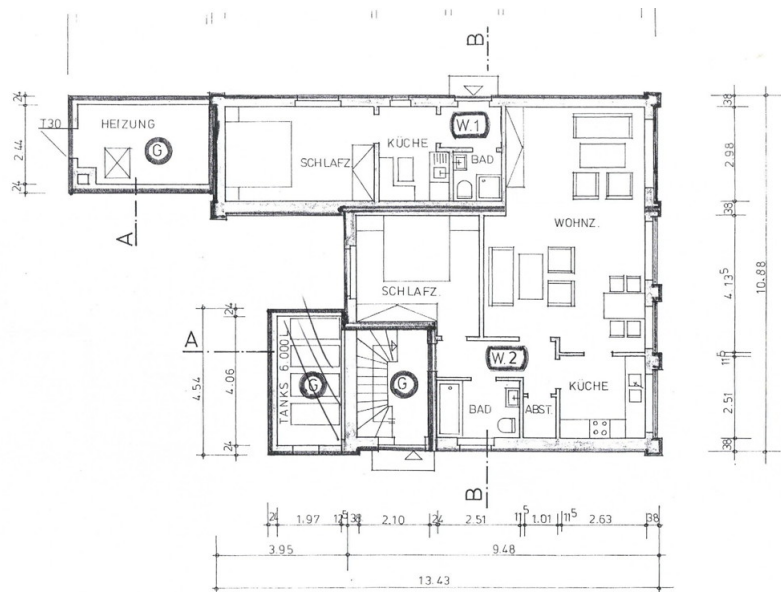
ERDGESCHOSS
