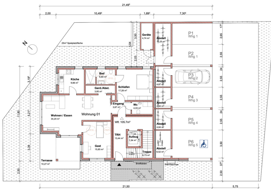
GRUNDRISS EG
