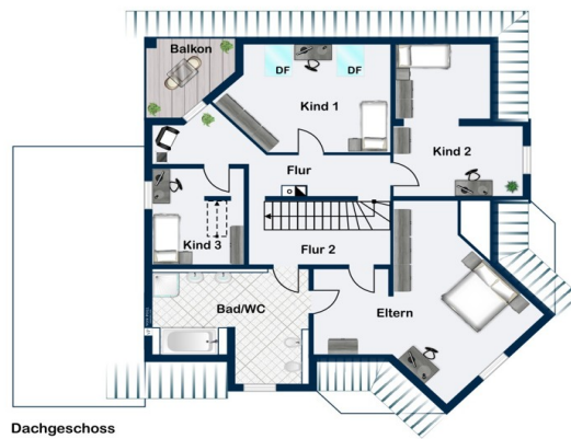
Dachgeschoss
