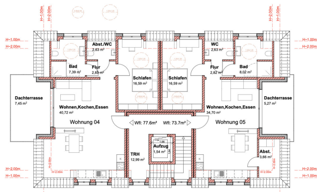
GRUNDRISS DG
