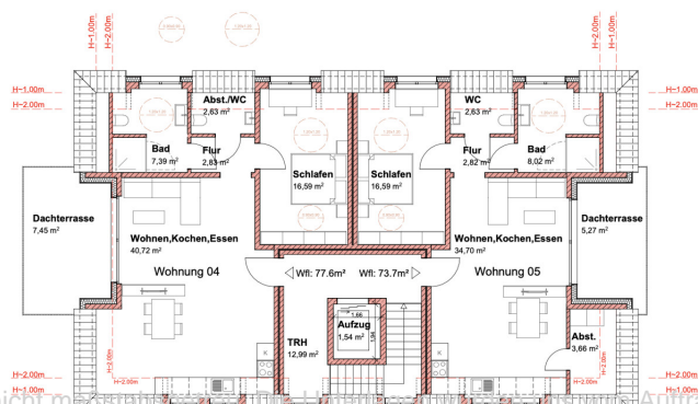
GRUNDRISS DG
