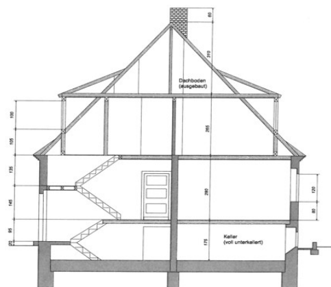
Querschnitt 1:50
