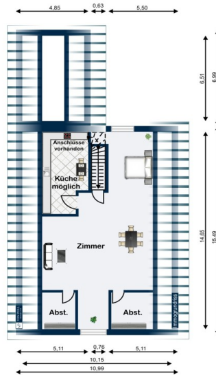
Dachgeschoss
