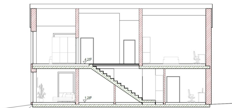
Schnitt C-C
