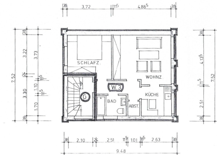
I. OBERGESCHOSS
