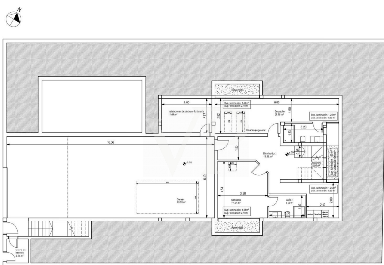
PLANTA SOTANO
