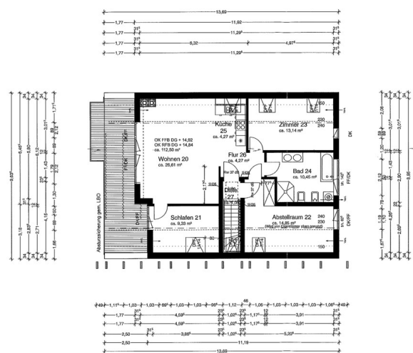
Grundriss DG
