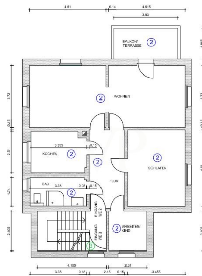
GRUNDRISSE OBERGESCHOSS
