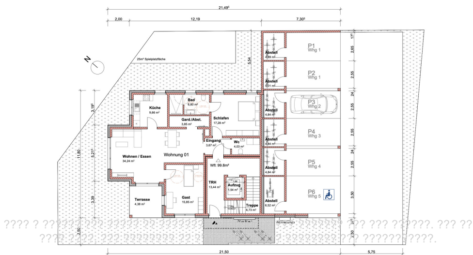
GRUNDRISS EG
