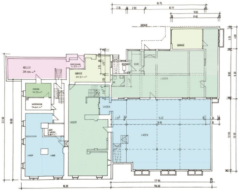
GRUNDRISS UNTERGESCHOSS M: 1:100
