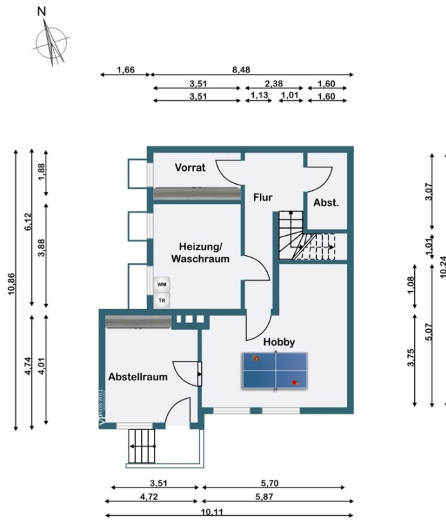
Kellergeschoss
