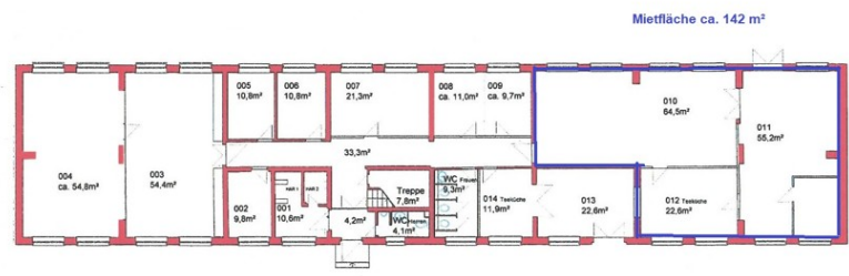
Grundriss Erdgeschoss
