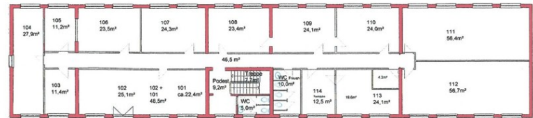
Grundriss Obergeschoss
