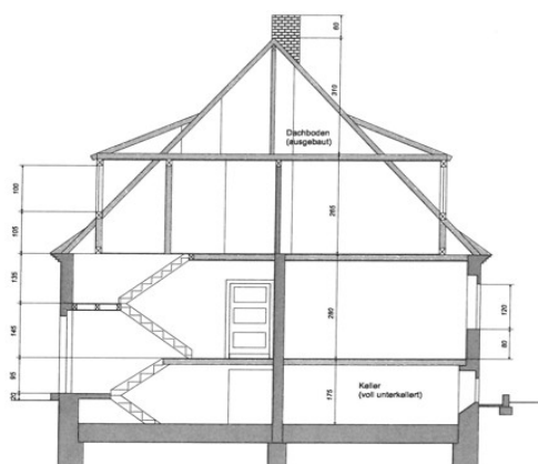
Querschnitt 1 : 20
