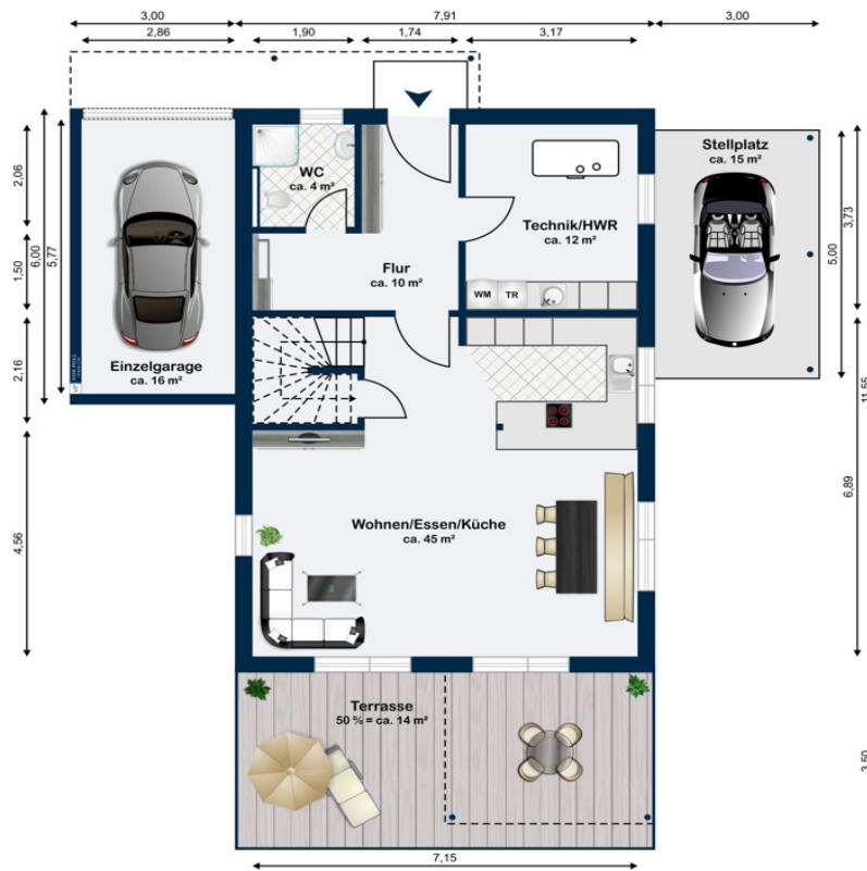
Erdgeschoss
