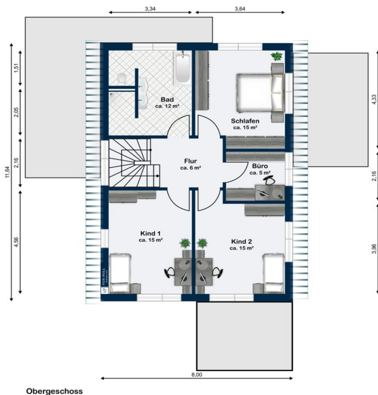
Obergeschoss
