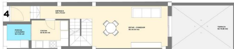
PLANTA PISO
