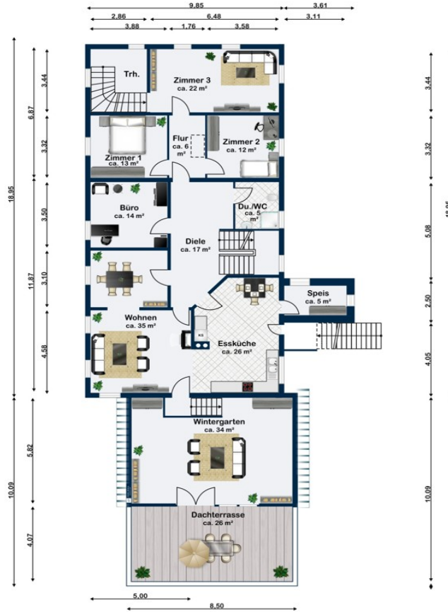
Obergeschoss
