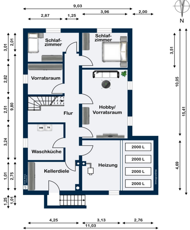
Kellergeschoss
