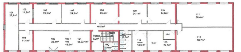
Grundriss Obergeschoss
