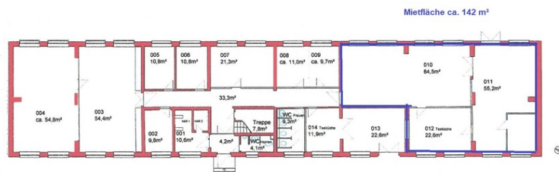
Grundriss Erdgeschoss
