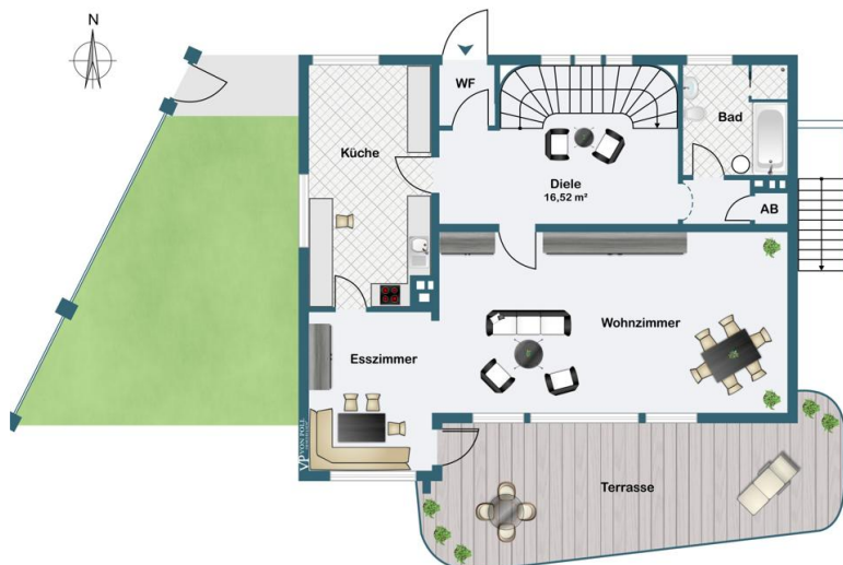
Erdgeschoss
