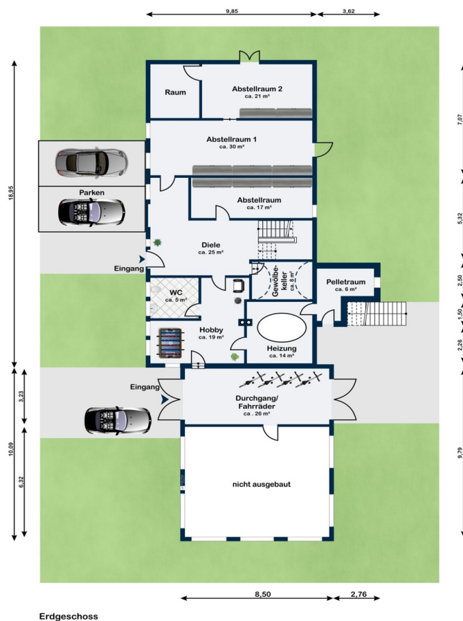
Erdgeschoss
